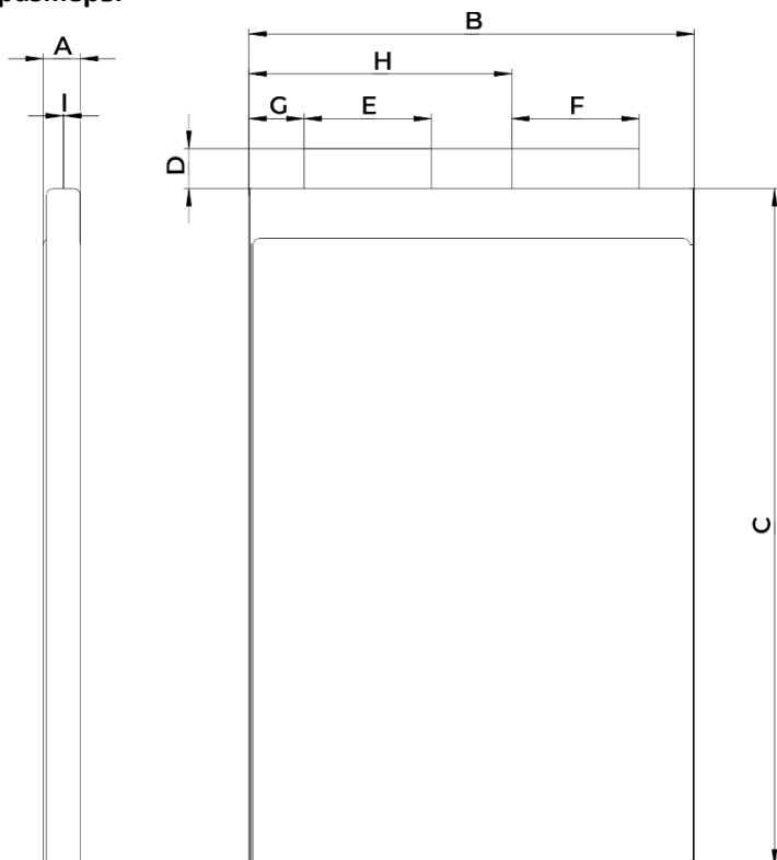
Рисунок 1 – Габаритные размеры LP1190190-30000
