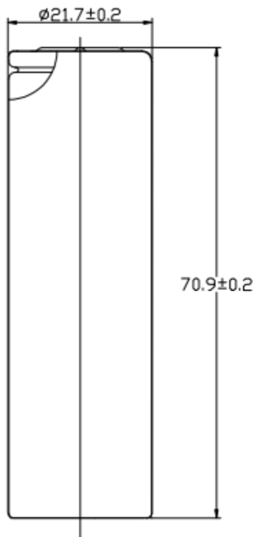
Рисунок 1 – Габаритные размеры LI21700-5000SE
