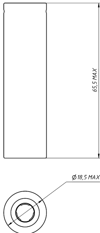
Рисунок 1 – Габаритные размеры LI18650T40-3000
