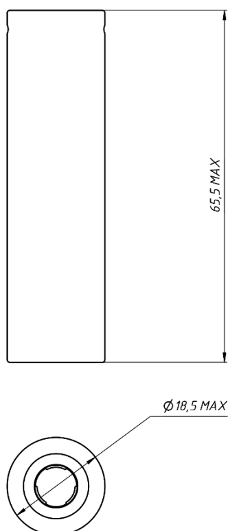
Рисунок 1 – Габаритные размеры LI18650T40-2800
