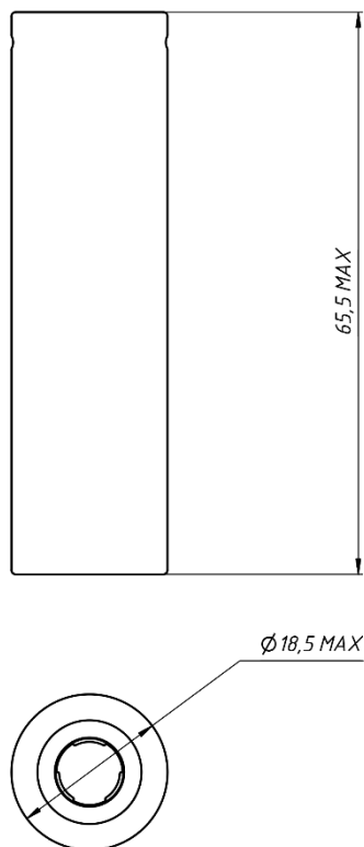
Рисунок 1 – Габаритные размеры LI18650-3000
