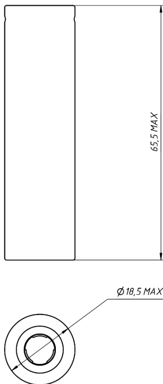
Рисунок 1 – Габаритные размеры LTO18650-1500CB
