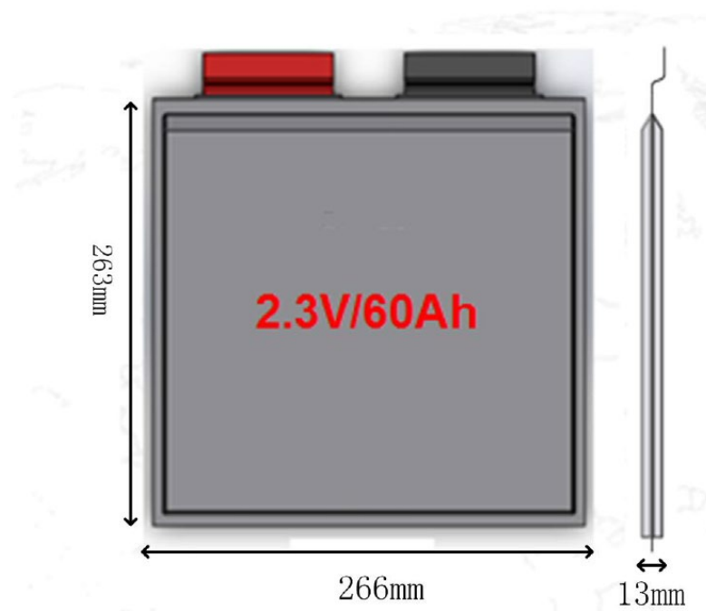
Рисунок 1 – Габаритные размеры
