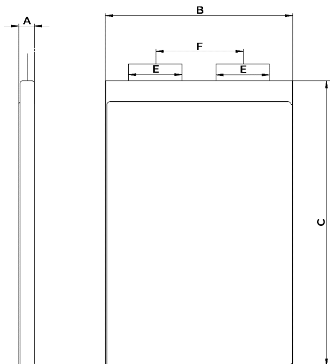
Рисунок 1 – Габаритные размеры LP9070170-12000
