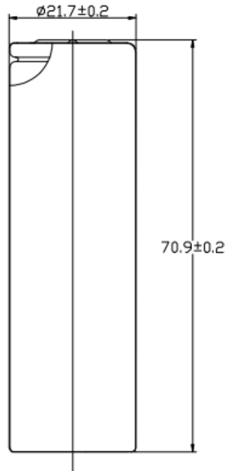
Рисунок 1 – Габаритные размеры LI21700-4000L
