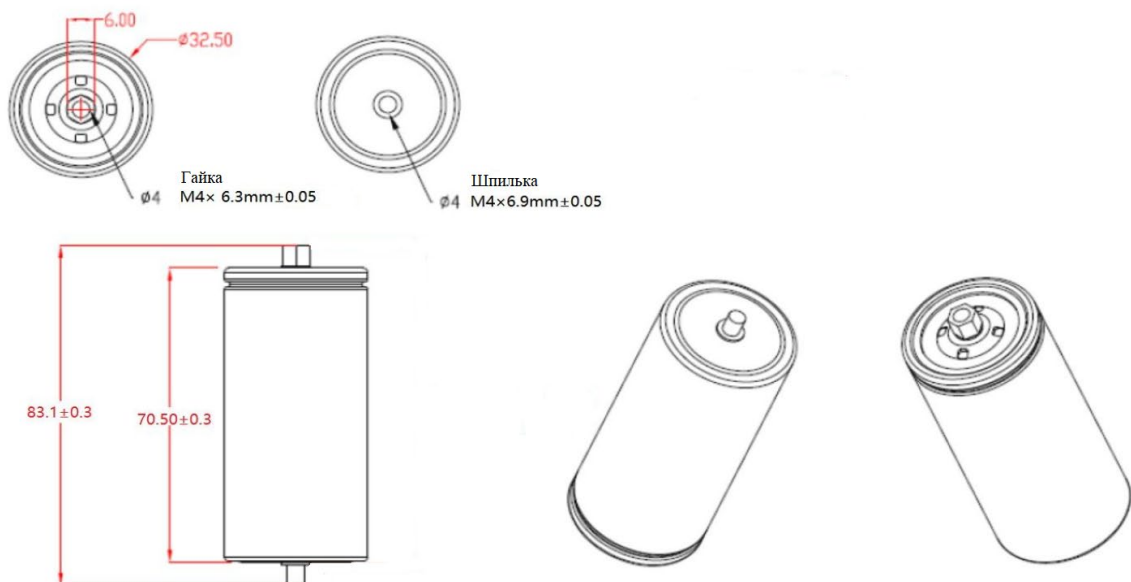
Рисунок 1 – Габаритные размеры LFP32700-6000PG
